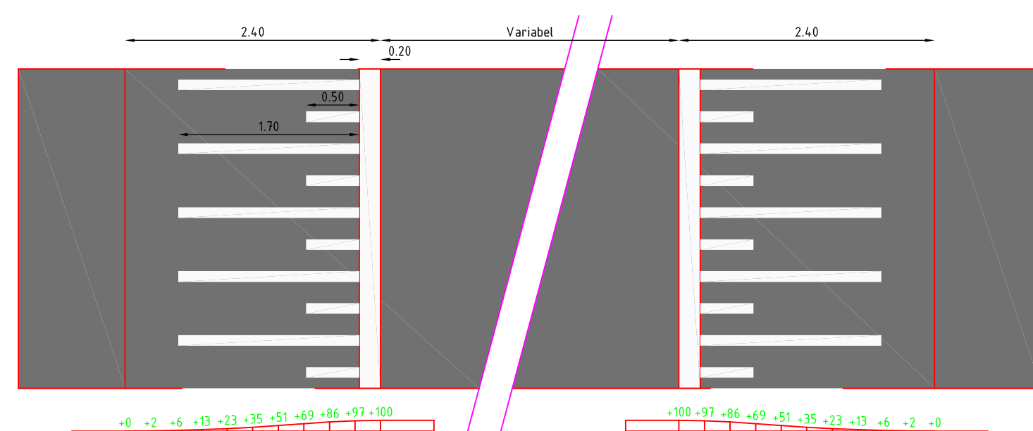
Detail kruispuntplateau
