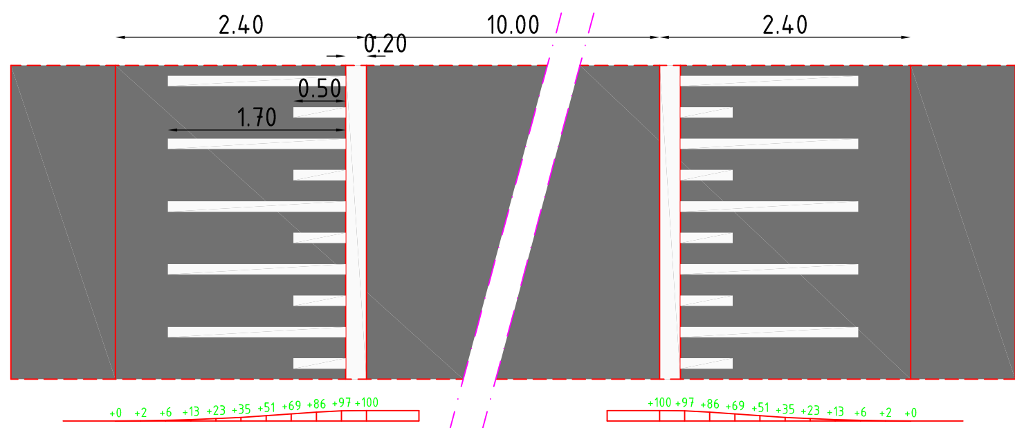
Detail d'empelplateau
