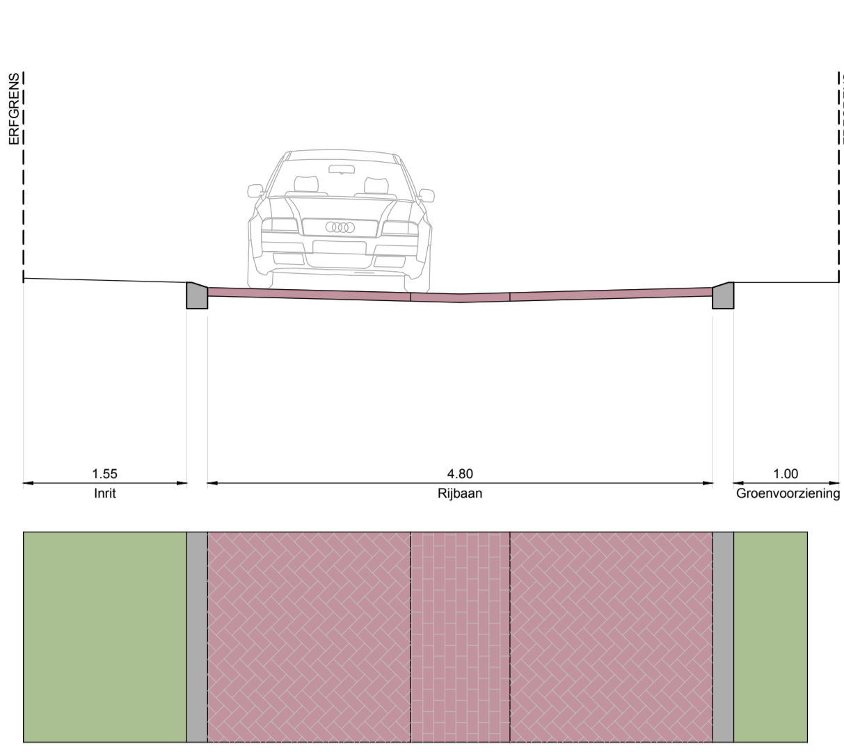
Dwarsprofiel B - B Situering: Schaal 1:50
