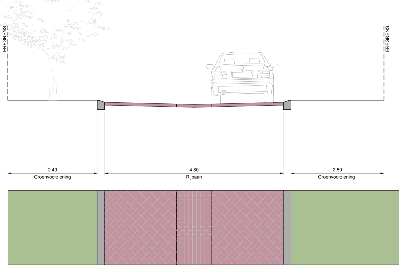
Dwarsprofiel A - A Situering: Schaal 1:50
